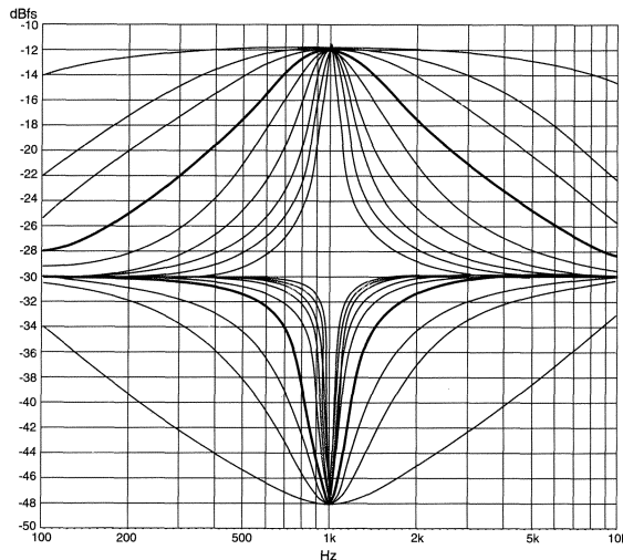
MPX 1 Parametric EQ: Q
